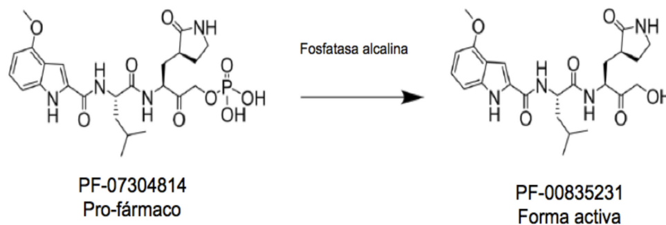
Figura 2 Activación por parte de las fosfatasa alcalinas celulares del pro-fármaco PF-07304814 a su forma activa PF-07321332 (nirmatrelvir).
